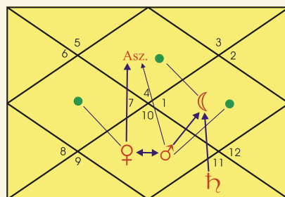
Das Beziehungsnetz des Aszendenten – hier zeigt sich die klare Struktur der SVA
