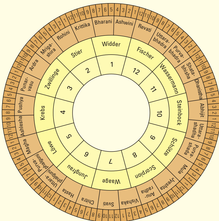
Das Rad mit den 12 Tierkreiszeichen, den 27 Nakshatras und den 108 Navamsas zeigt in übersichtlicher Weise die komplexen Zusammenhänge der vedischen Astrologie
