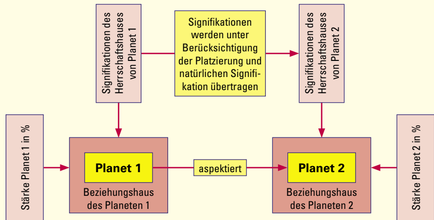
Das Beziehungsdiagramm zwischen zwei Planeten
